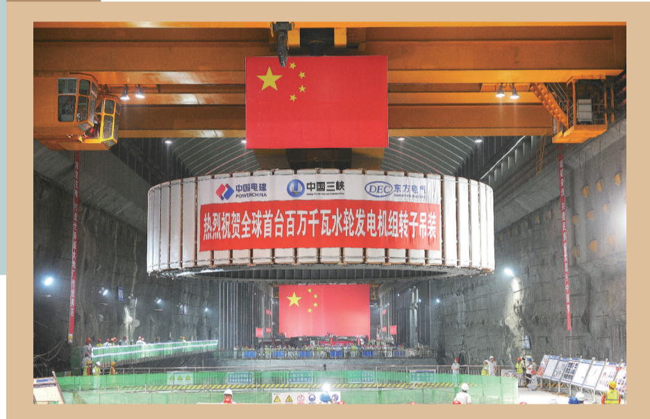
由东方电机自主研发的全球首台百万千瓦水轮发电机组转子在白鹤滩水电站成功吊装。
